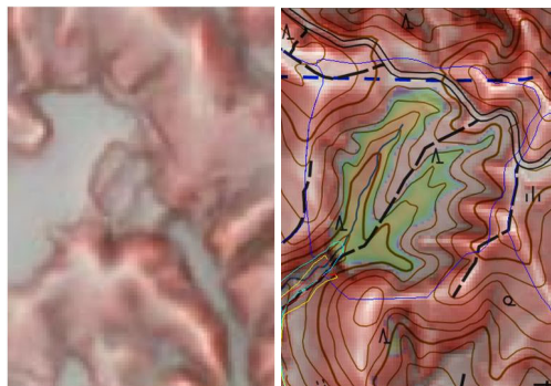
(左) 谷埋め盛土造成中箇所5mメッシュDEMによる赤色立体地図 (右) 谷埋め盛土箇所の5mメッシュDEMと10mメッシュDEMの標高差解析例
