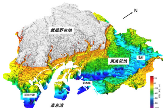
東京低地の地下の埋設谷形状
