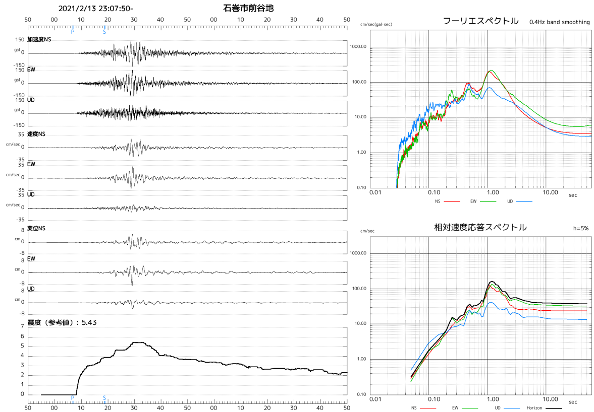
図2 強震観測データ【石巻市前谷地】
