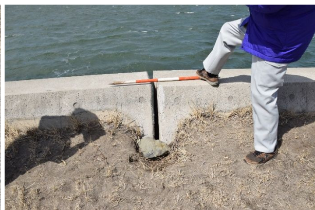
護岸の変状および護岸背面地盤の亀裂 ※噴砂は確認できず
