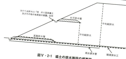
雨水 図 V・2-1 盛土の排水施設の概要
